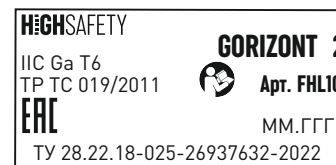
Рис. 2 Маркировка элементов анкерной линии GORIZONT 2.
